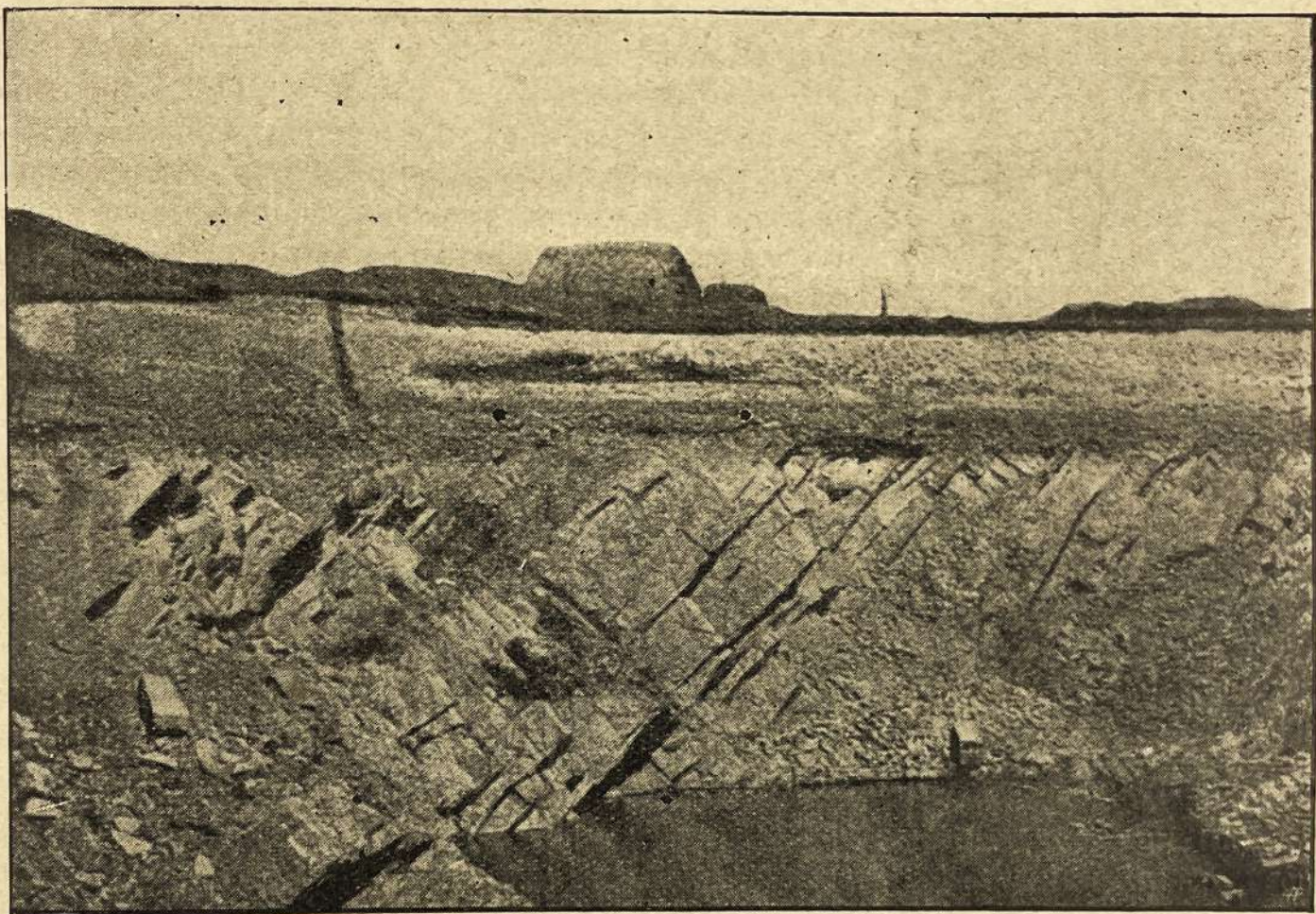
Fig. 114. — Stratificazione discordante tra calcari orizzontali e quarziti inclinate a May nel Calvados.
