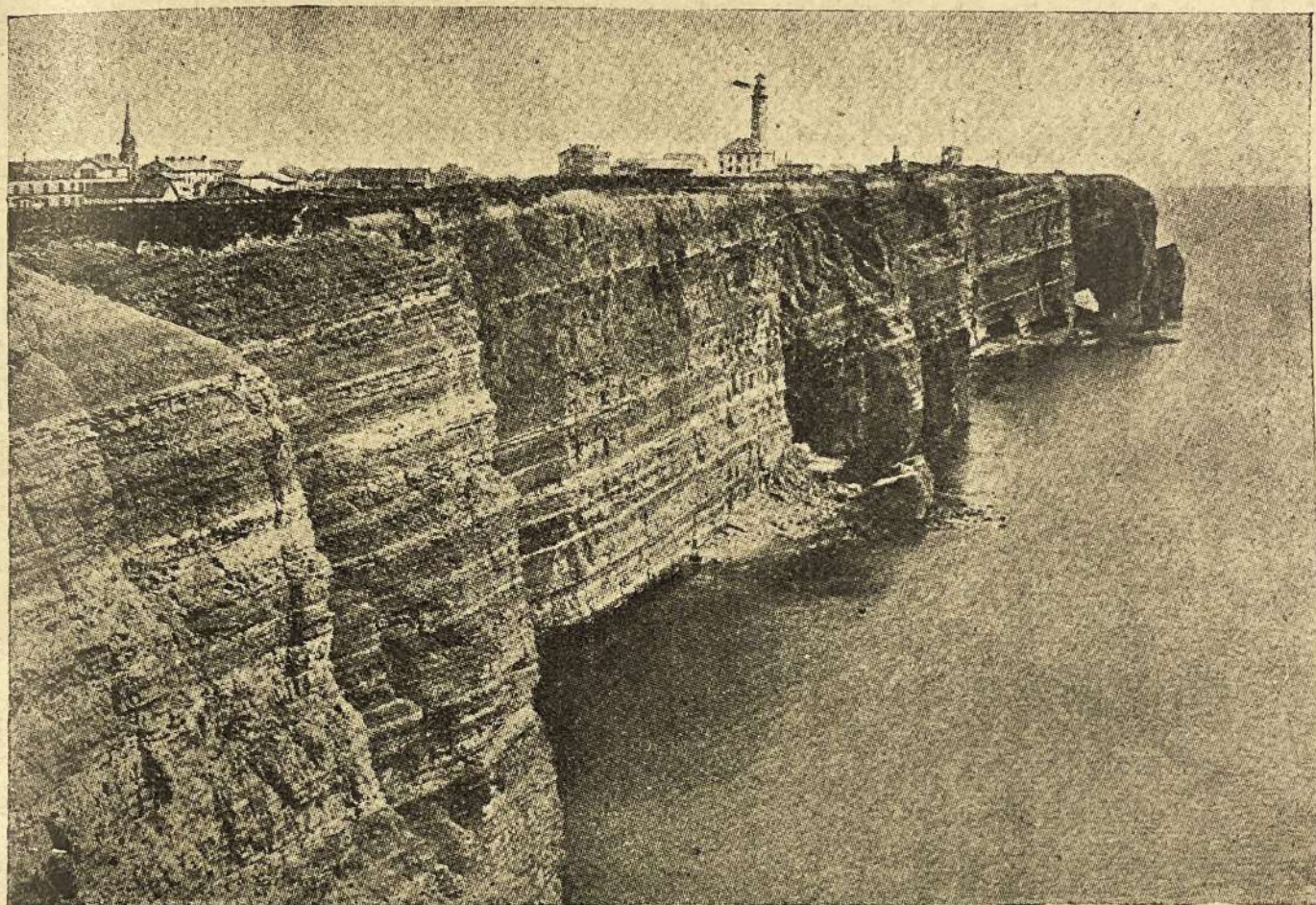
Fig. 58. — Costiera a stratificazione regolare di Helgoland.
